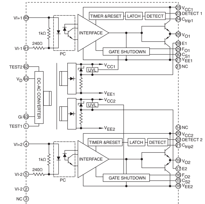
VLA567-01R
