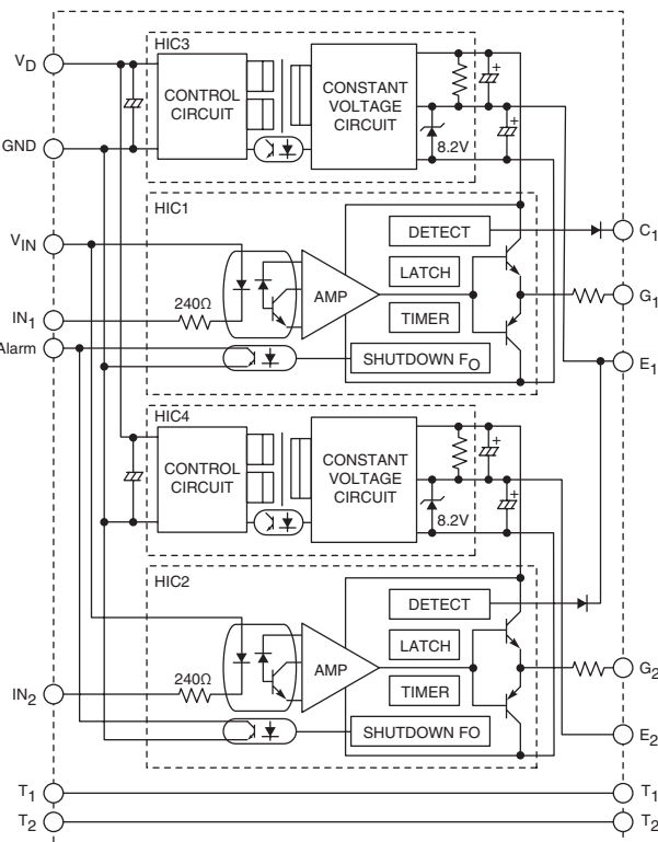
VLA536-01R
