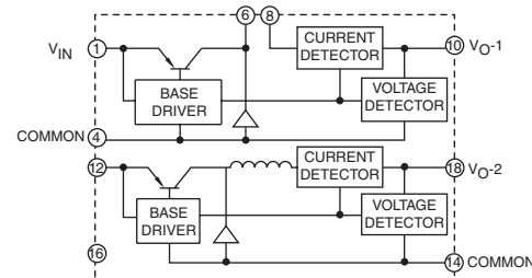
M57184N-715B
