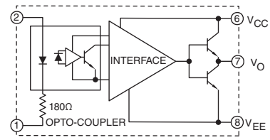
VLA507-01, VLA513-01
