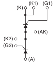
PA43--06, PA43--07
